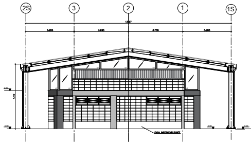
VISTA 04 ESC.: 1.50
