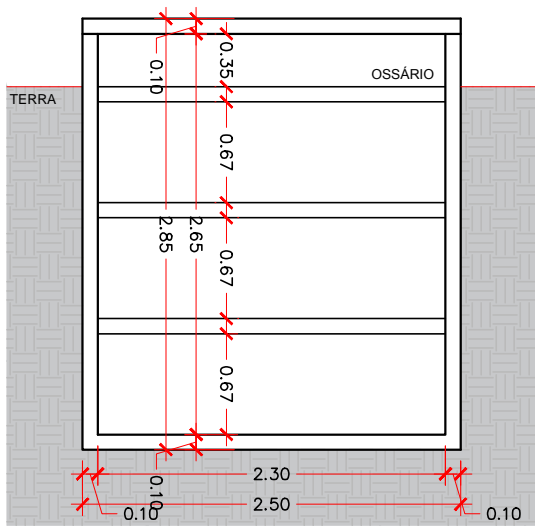
CORTE B-B TÚMULO (TIPO FAMILIAR) ESC.: 1:50
