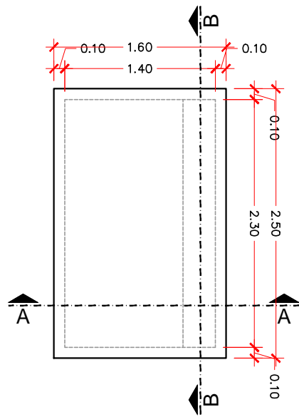
PLANTA BAIXA TÚMULO (TIPO FAMILIAR) ESC.: 1:50
