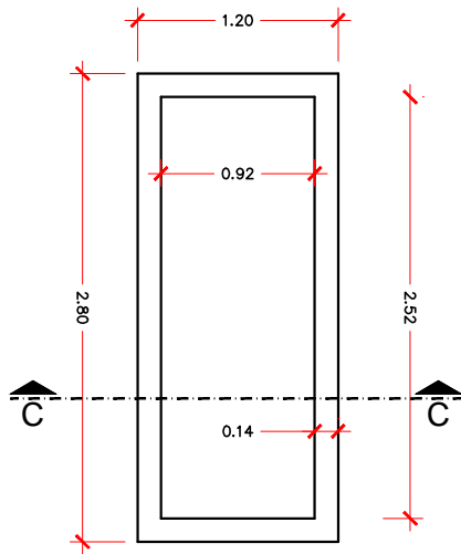
PLANTA BAIXA TÚMULO (TIPO ROTATIVO) ESC.: 1:50
