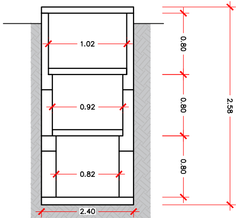
CORTE C-C TÚMULO (TIPO ROTATIVO) ESC.: 1:50
