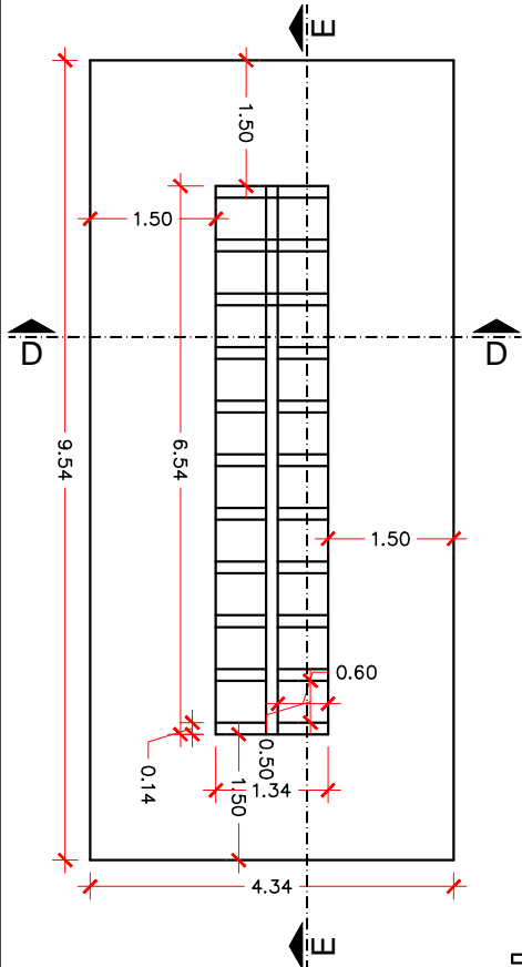
PLANTA BAIXA OSSUÁRIO ESC.: 1:100
