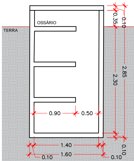
CORTE A-A TÚMULO (TIPO FAMILIAR) ESC.: 1:50
