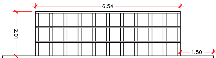
CORTE D-D OSSUÁRIO ESC.: 1:100
